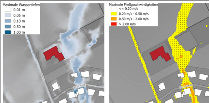
Abbildung 1: Maximale Wassertiefen und Fließgeschwindigkeiten im Bereich des Objekts
